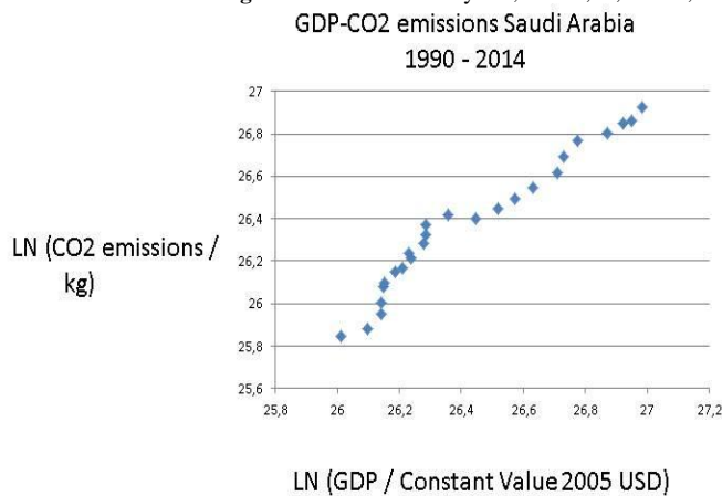
Figure-8. Saudia Arabia: y = 1,03x - 0,77 ; R^2 = 0,95
