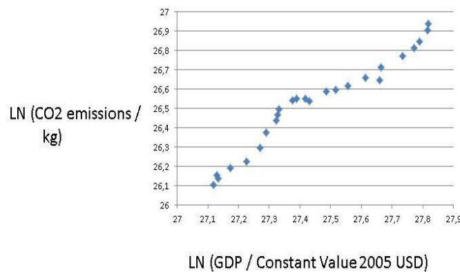
Figure-14. Brazil GDP-CO 2 : y = 1,03x - 1,7 ; R^2 = 0,95
